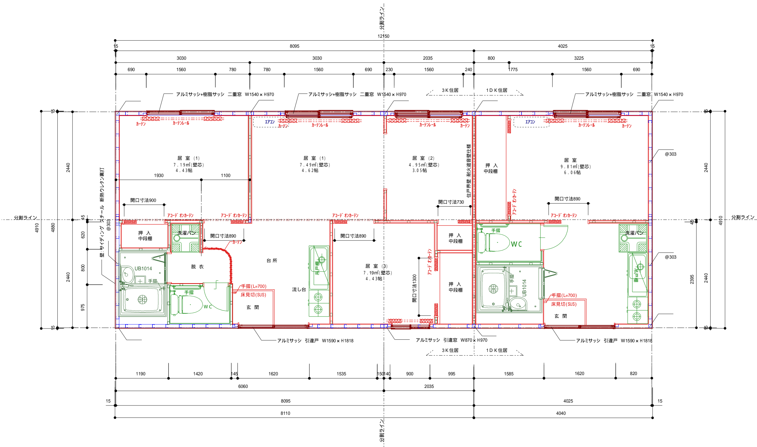
平面図 1:50
